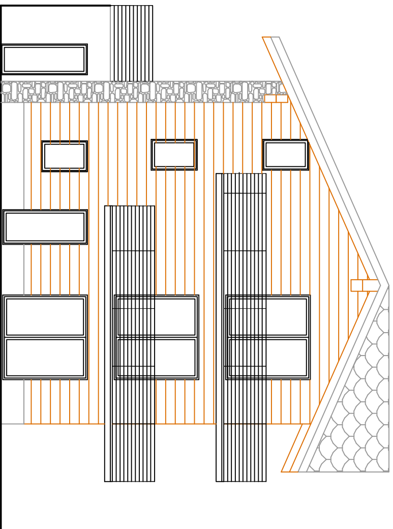
PROSPETTO OVEST
