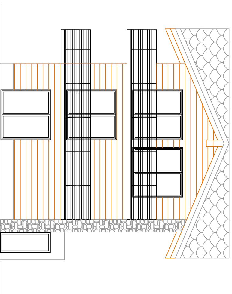
PROSPETTO SUD
