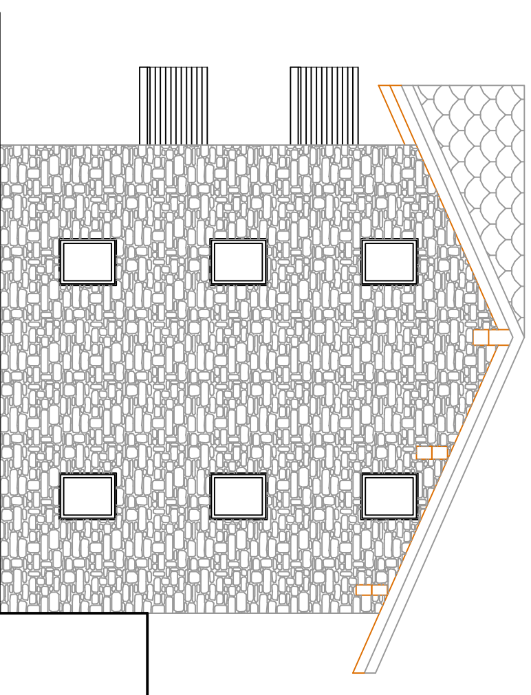
PROSPETTO EST
